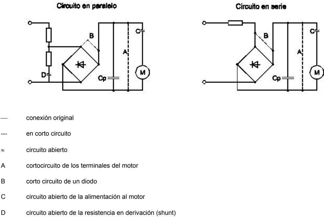
Figura F.1. Simulación de defectos
