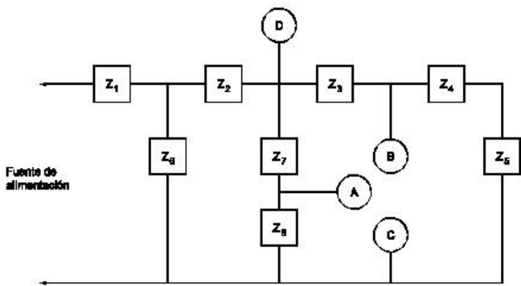
Figura 8. Diagrama para el ensayo de rigidez dieléctrica a la temperatura de operación
