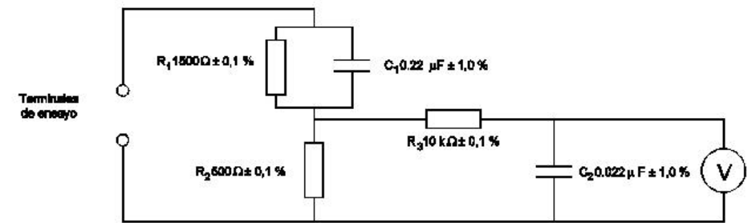
Figura G.1. Circuito para medir las corrientes de fuga
