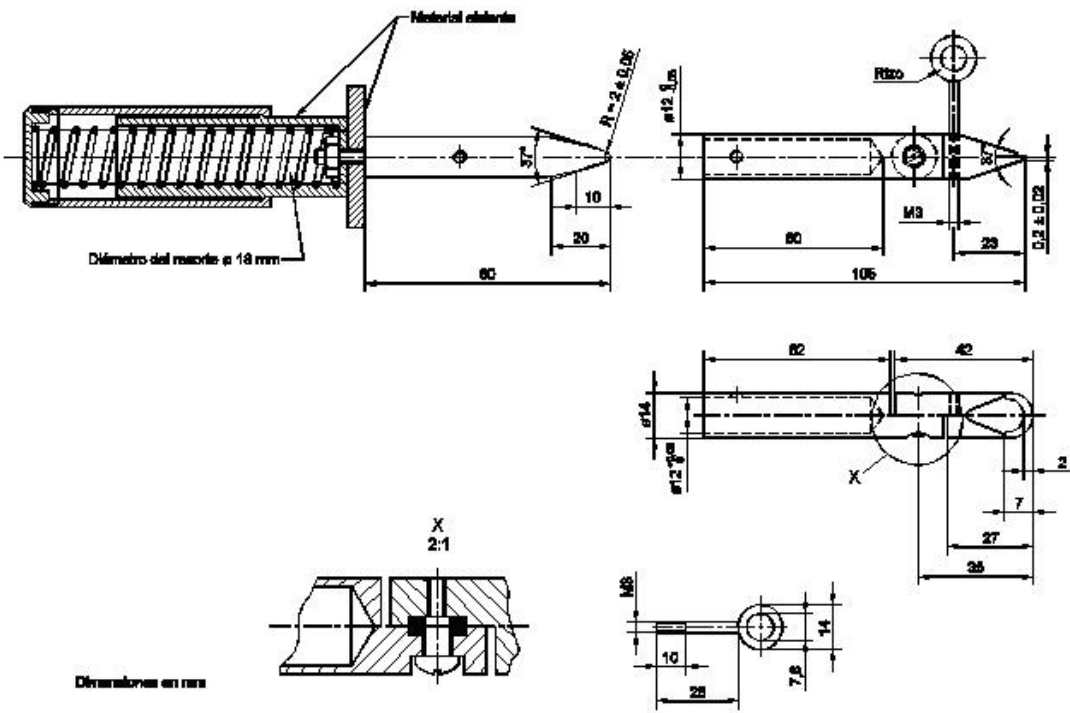
Figura 10. Uña de ensayo
